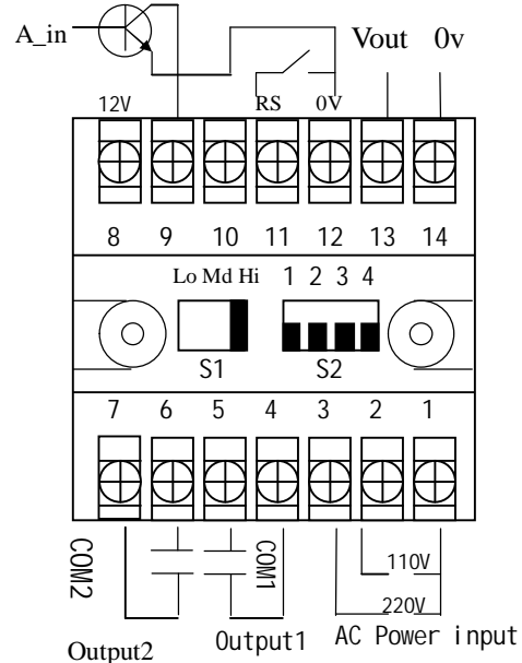
SC-62KE 端子说明。 Connection Diagram of SC-62KE
